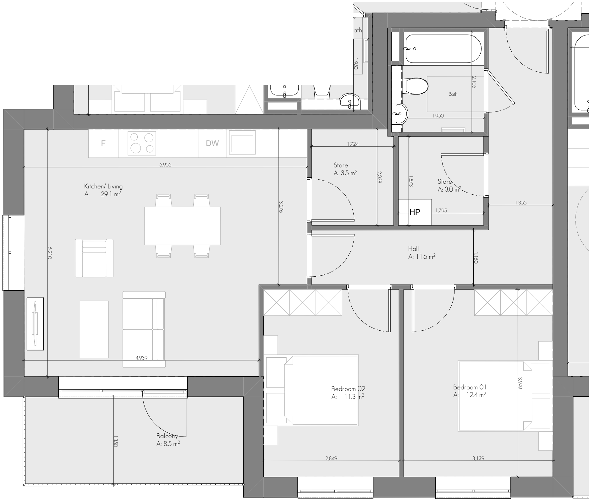
Apartment Type 2E 1:50
