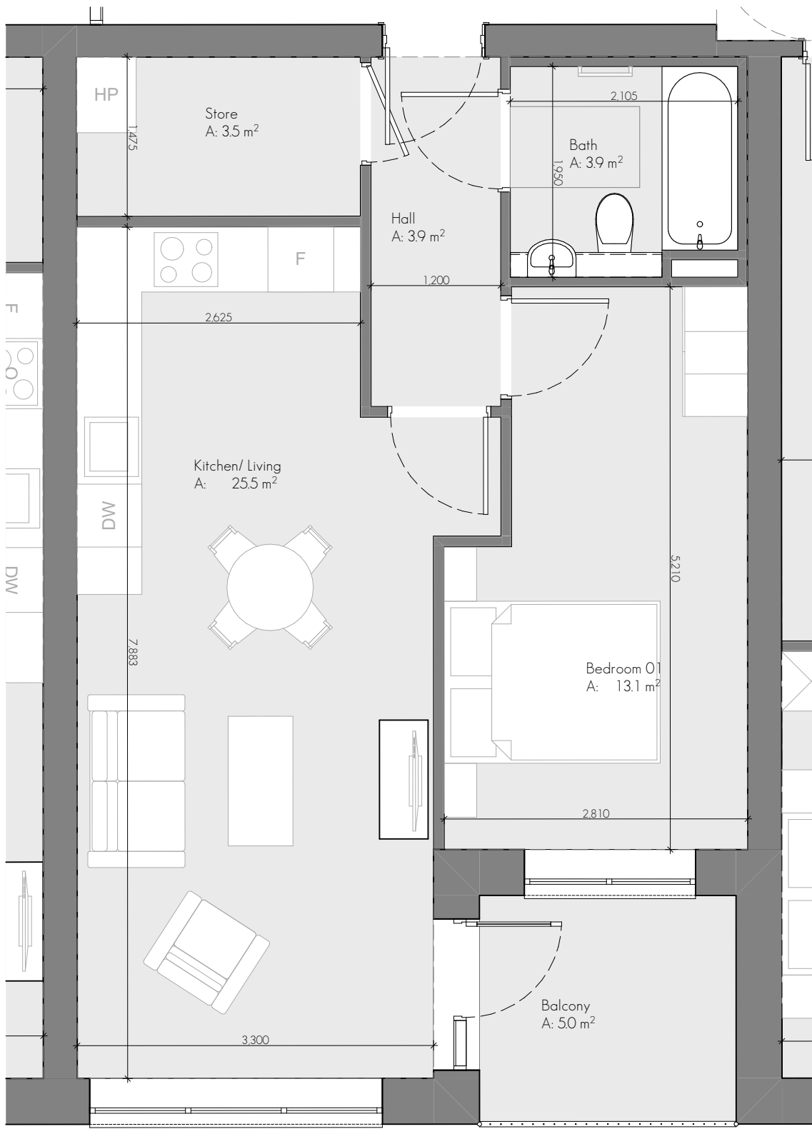
Apartment Type 1E 1:50
